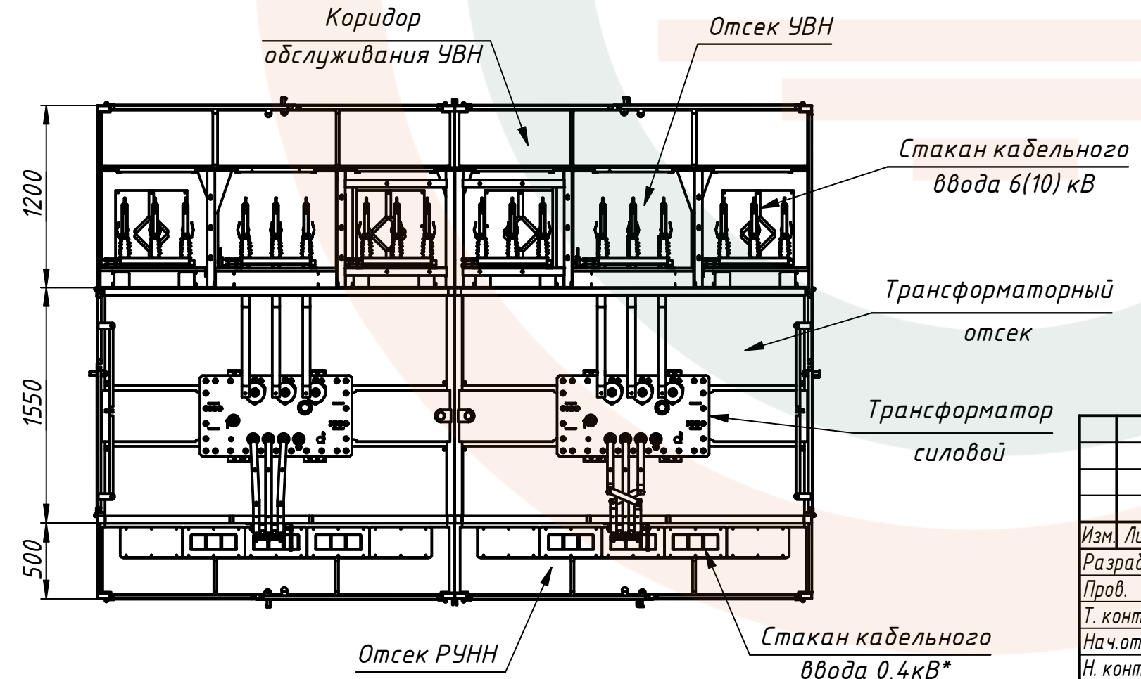
A-A (1:35)
