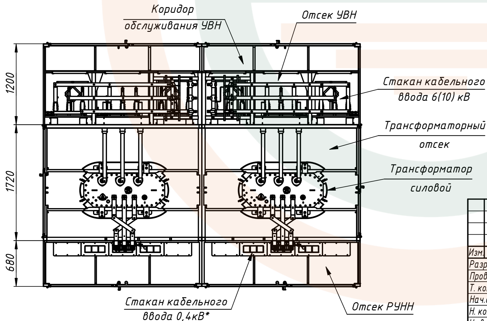
A-A (1:35)
