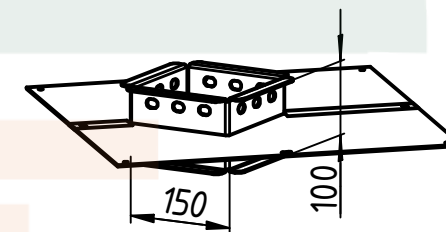
Стакан кабельного ввода 6(10)кВ
