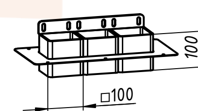
Стакан кабельного ввода 0,4кВ*
