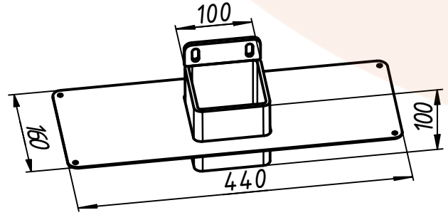
Стакан кабельного ввода 0,4кВ*
