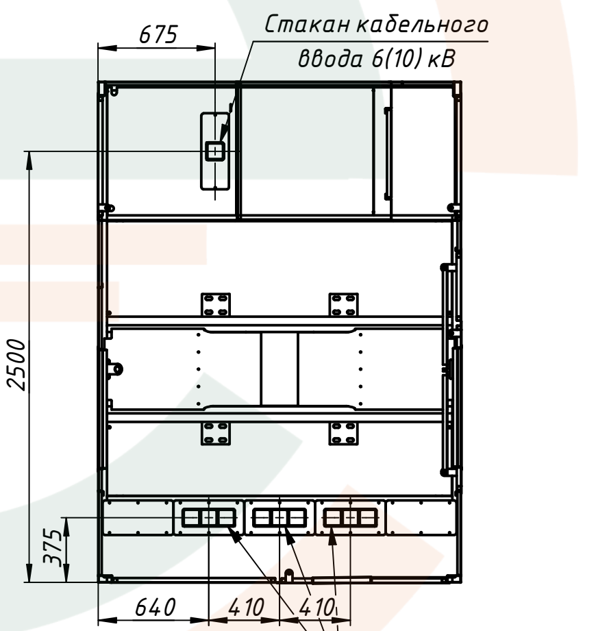
Б-Б План основания
