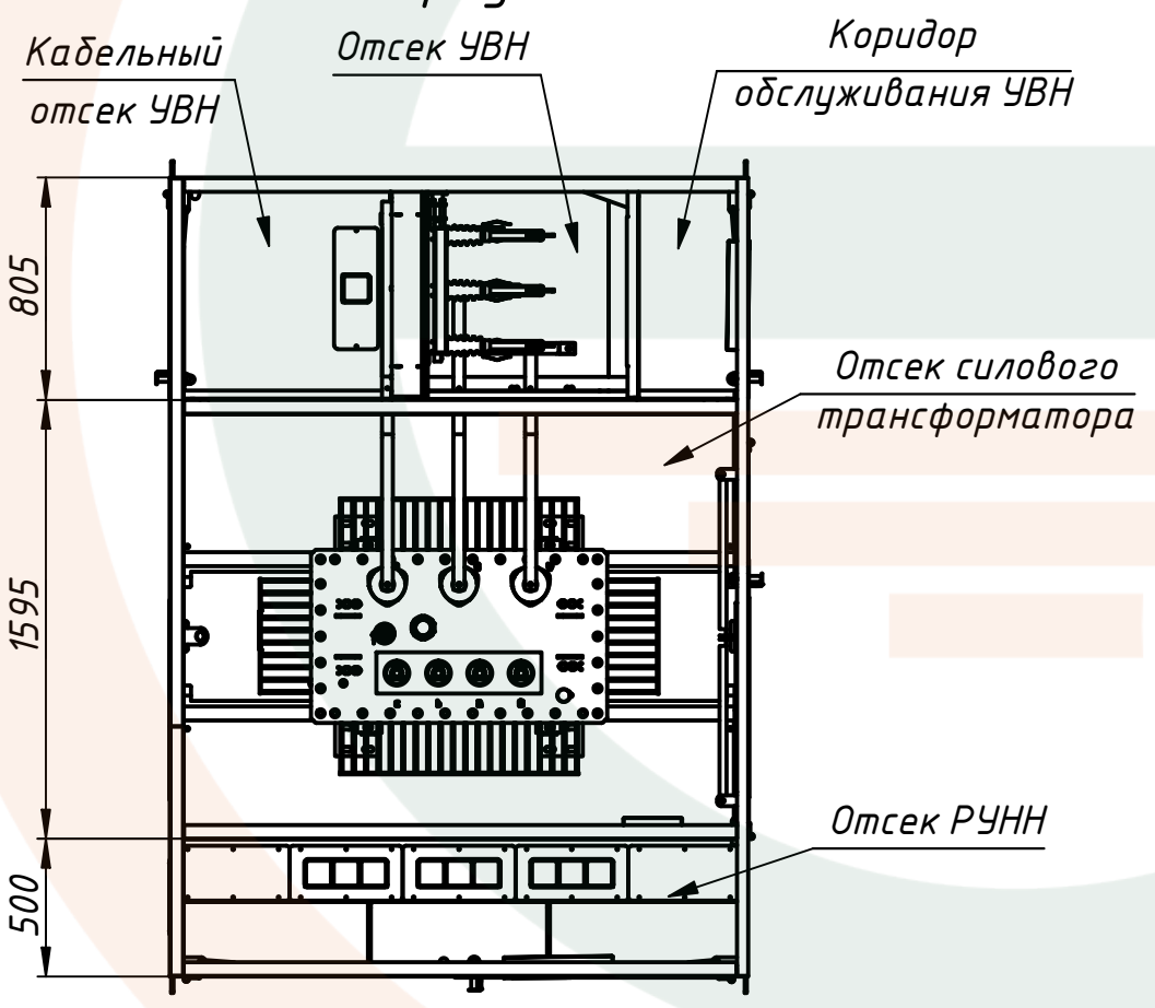
А-А повернуто
