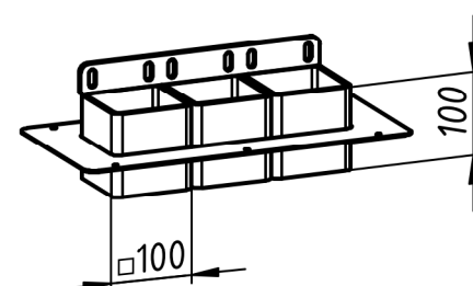
Стакан кабельного ввода 0,4 кВ*
