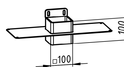
Стакан кабельного ввода 6(10) кВ
