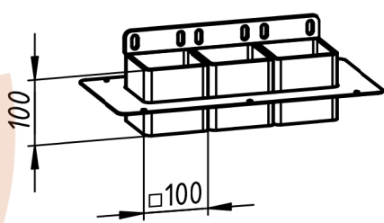
Стакан кабельного ввода 0,4кВ*
